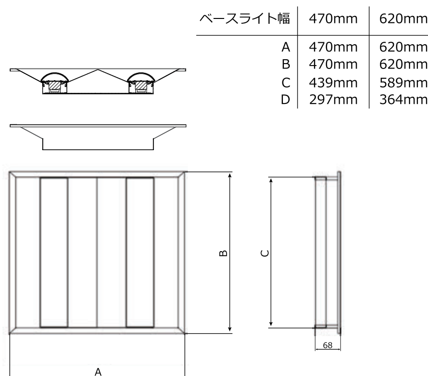
スクエアベースライト寸法詳細図
